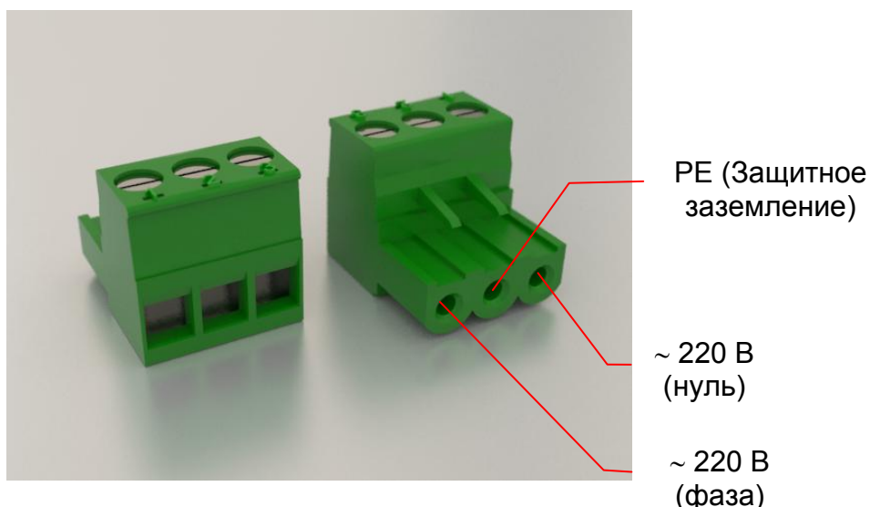
Рис. 2.4. Внешний вид разъема MSTB 2.5/3 и назначение контактов
