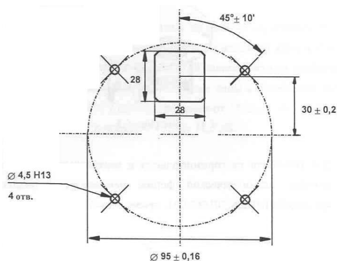
Рис.6.6. Внешний вид площадки для установки антенного блока
