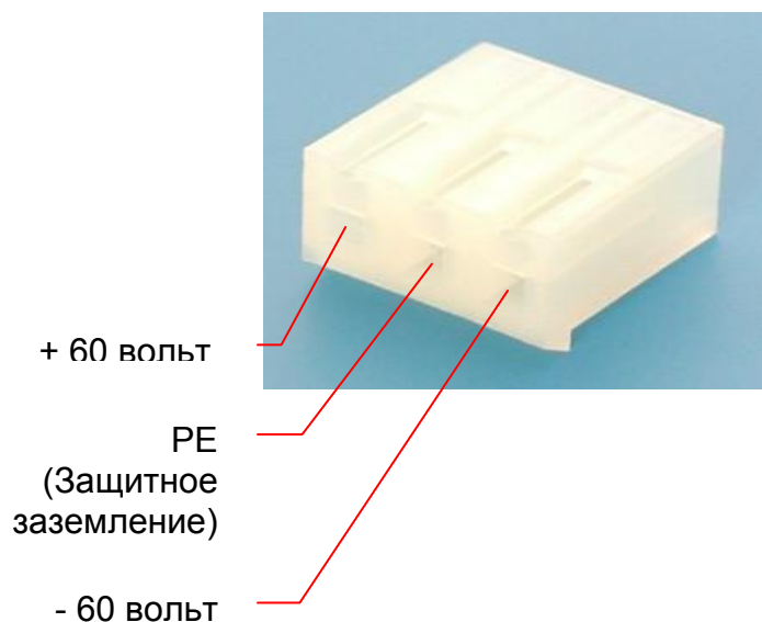
Рис. 2.3. Внешний вид разъема питания PNU-3 и назначение контактов
