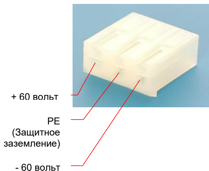
Рис. 2.3. Внешний вид разъема питания PDU-3 и назначение контактов
