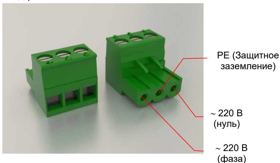
Рис. 2.4. Внешний вид разъёма MSTB 2.5/3 и назначение контактов
