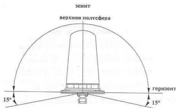
Рис.6.5. Верхняя полусфера антенны
