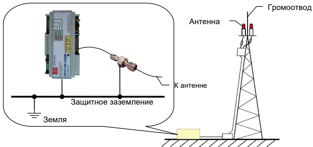
Рис.6.10. Пример установки защитного элемента
